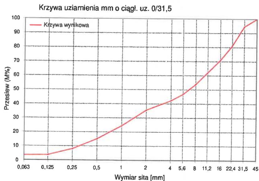
Rys. 1 Wykres krzywej uziarnienia - próbka TPA/WK/20/0923
