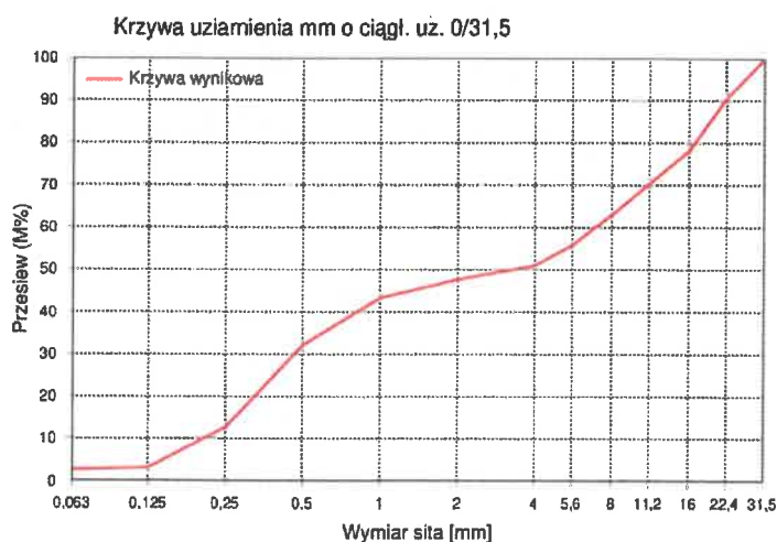
Rys. 1 Wykres krzywej uziarnienia - próbka TPA/WK/20/0922
