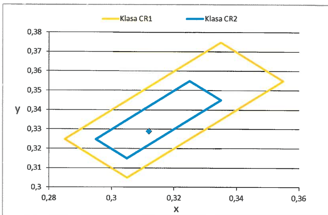
Wykres 1. Wykres współrzędnych chromatyczności x, y – pole barwy białej.
